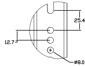
細部B 縮尺1:8
