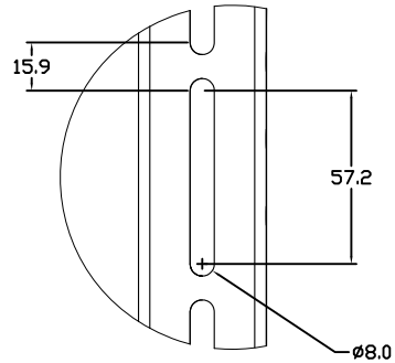
細部A 縮尺1:8
